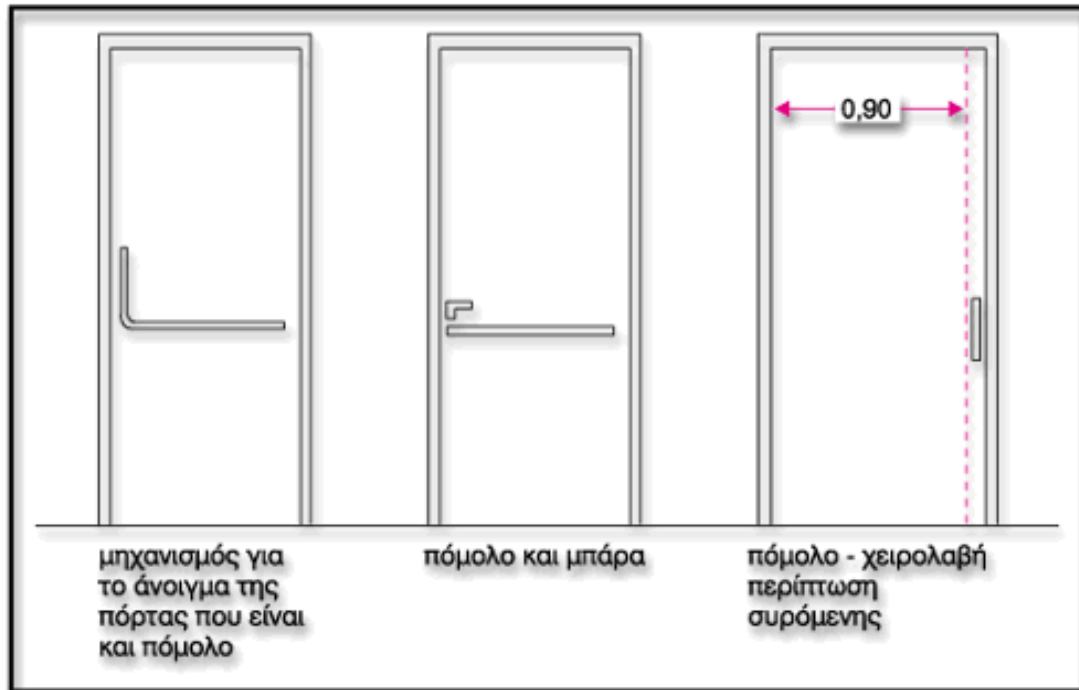
Σχήμα 3: Πόρτα εξόδου χώρων υγιεινής
