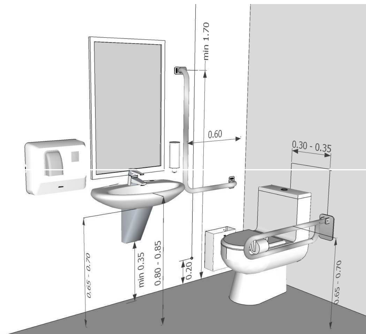
Σχήμα 4: Ενδεικτική διάταξη χώρου υγιεινής Α.Μ.Ε.Α.
